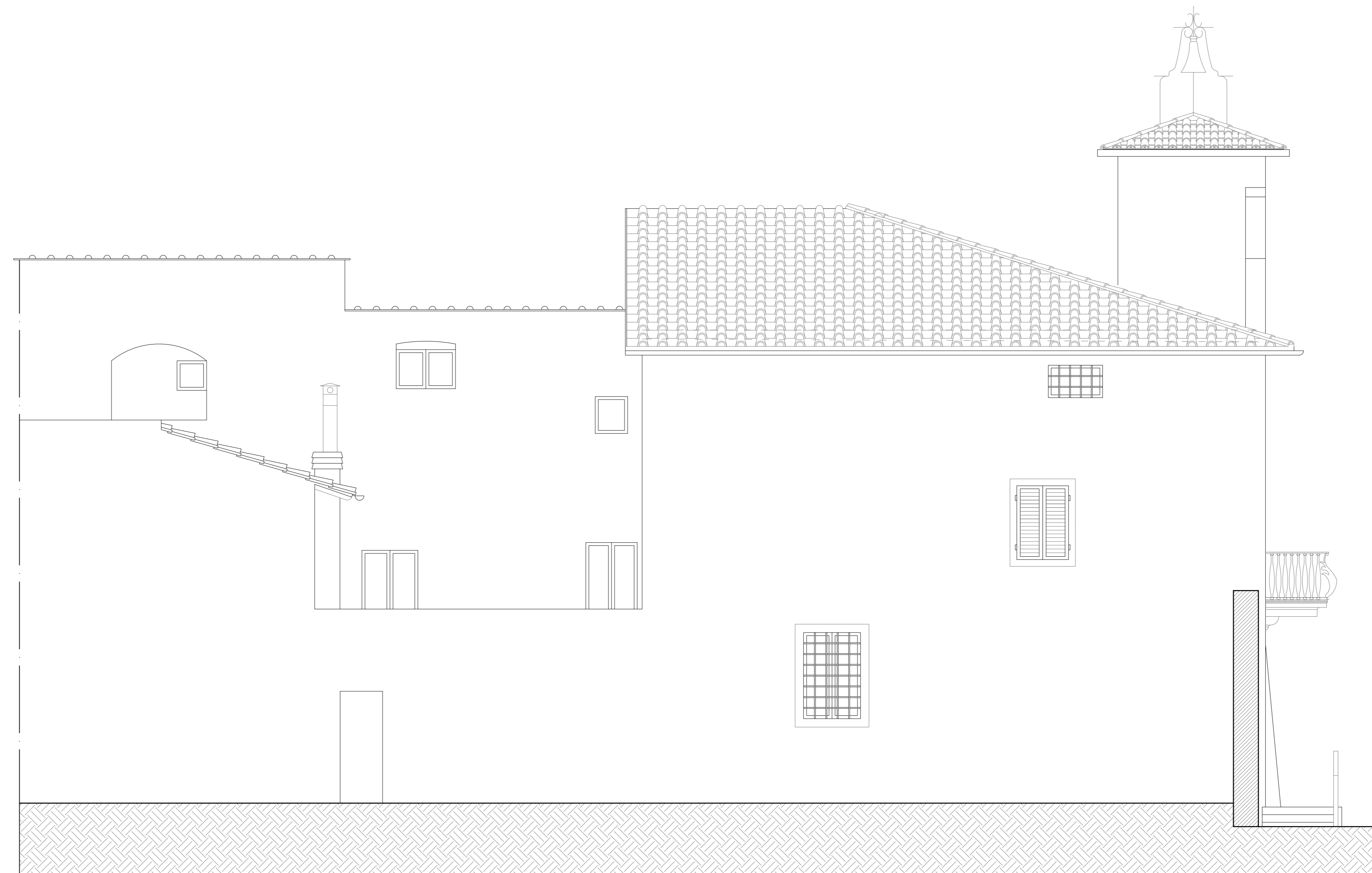
STATO ATTUALE - PROSPETTO NORD-EST SCALA 1:50
