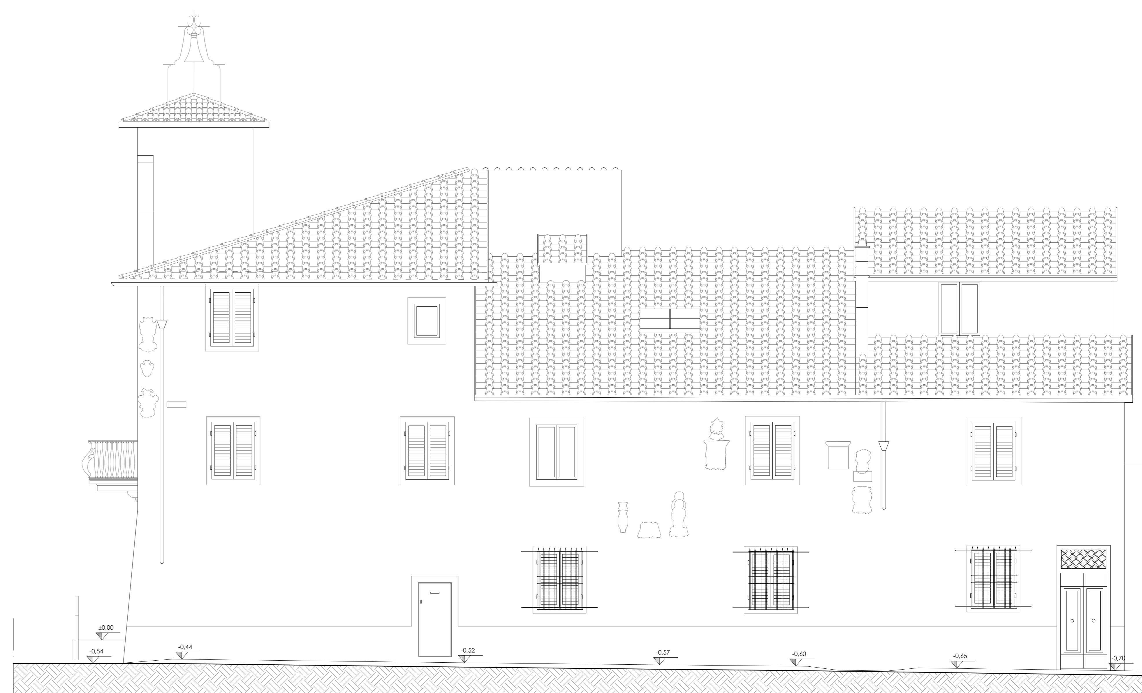
STATO ATTUALE - PROSPETTO SUD-OVEST SCALA 1:50
