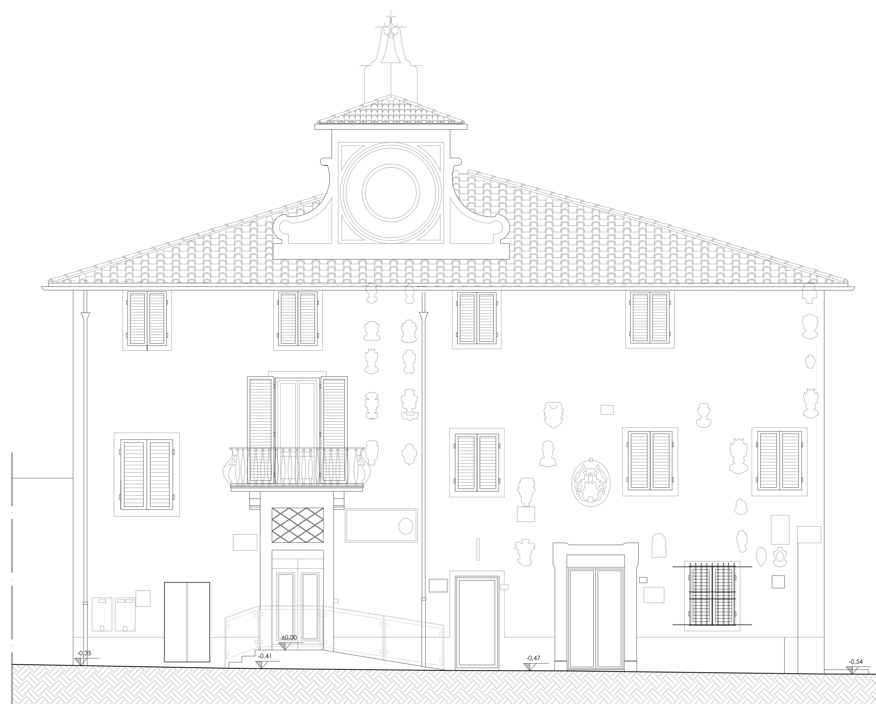
STATO ATTUALE - PROSPETTO NORD-OVEST SCALA 1:50
