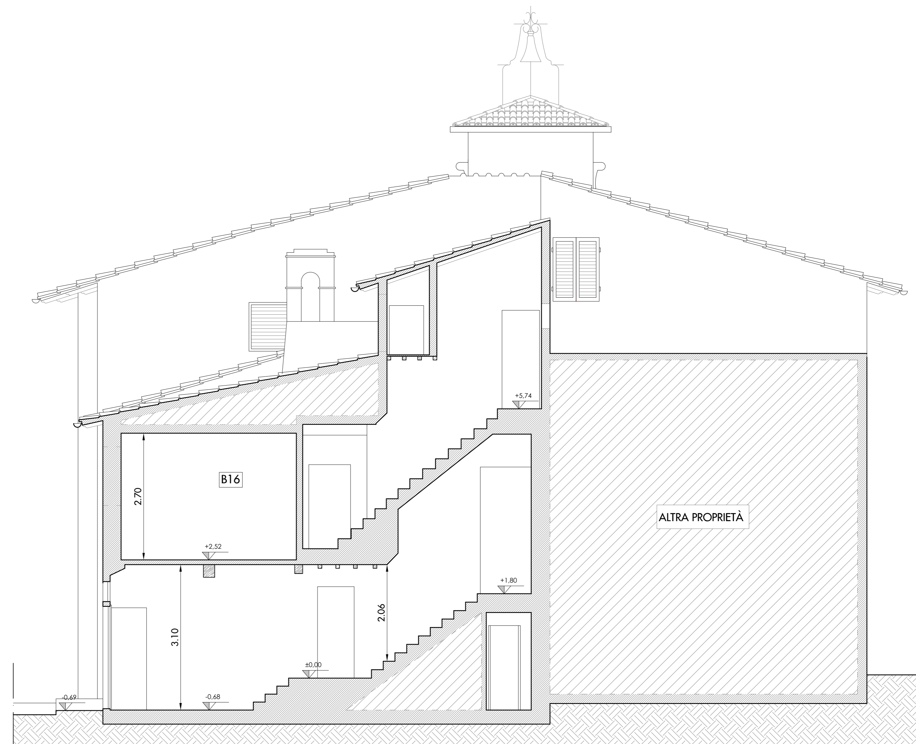
STATO ATTUALE - SEZIONE CC' SCALA 1:50
