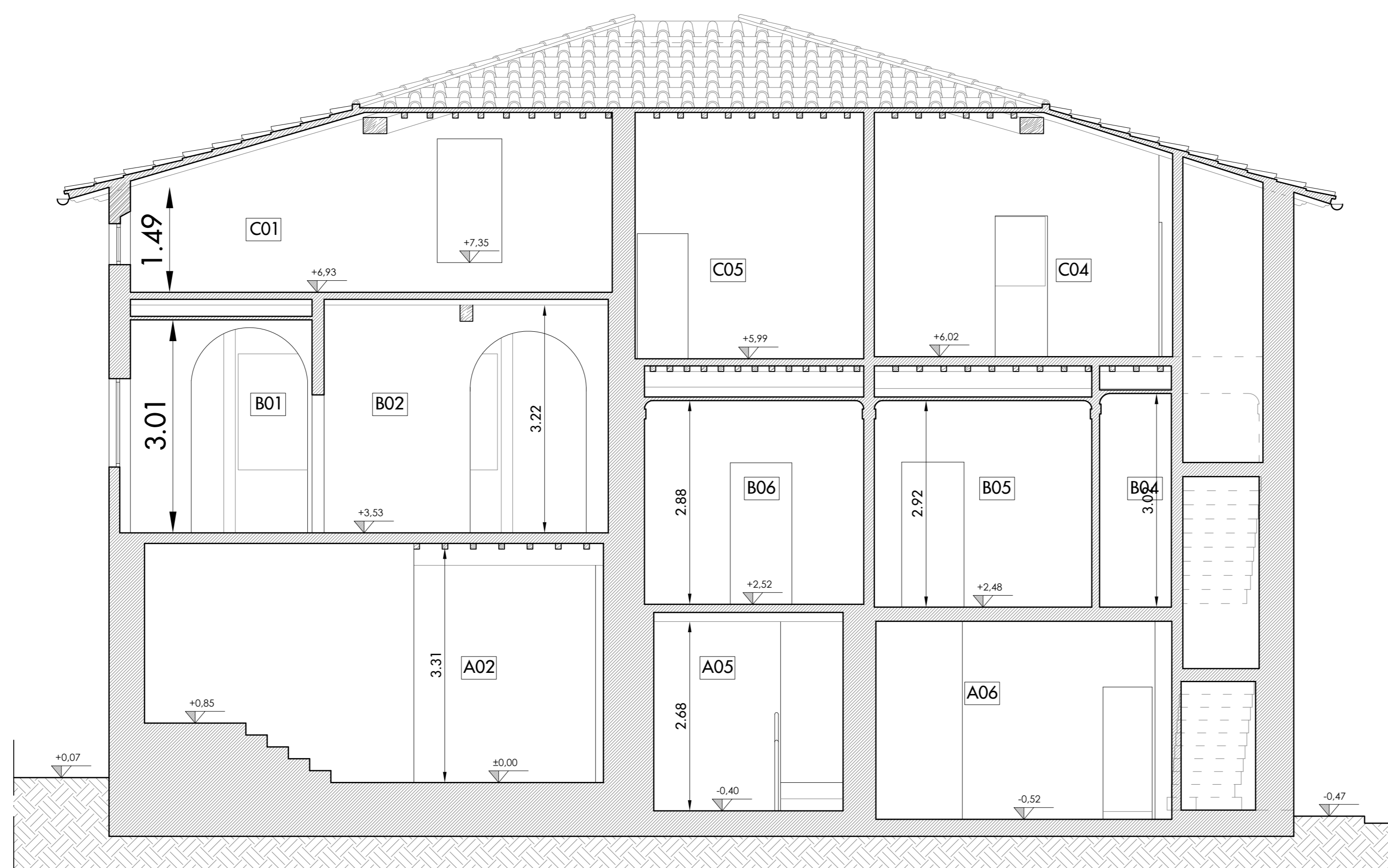
STATO ATTUALE - SEZIONE AA' SCALA 1:50
