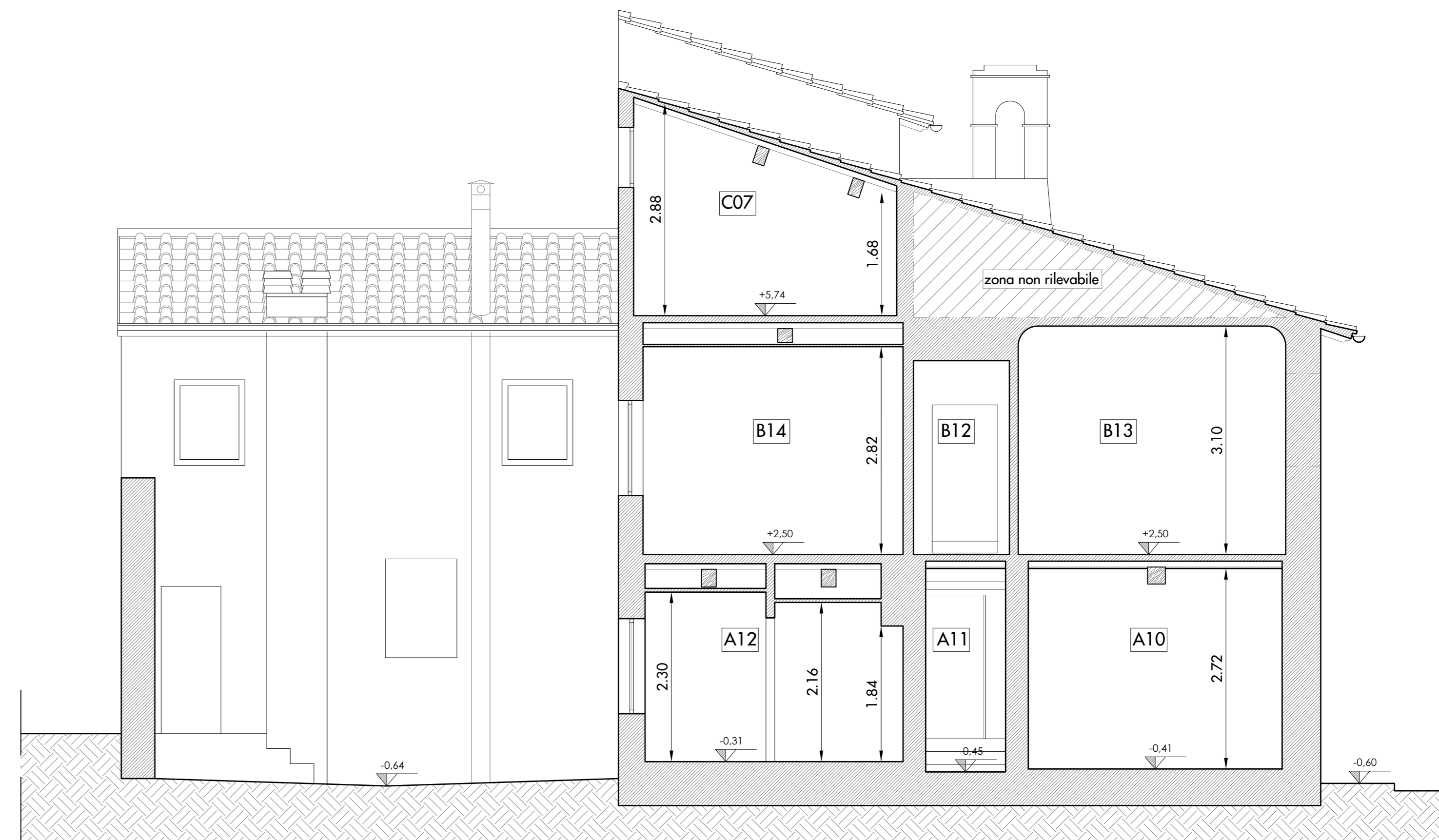
STATO ATTUALE - SEZIONE BB' SCALA 1:50
