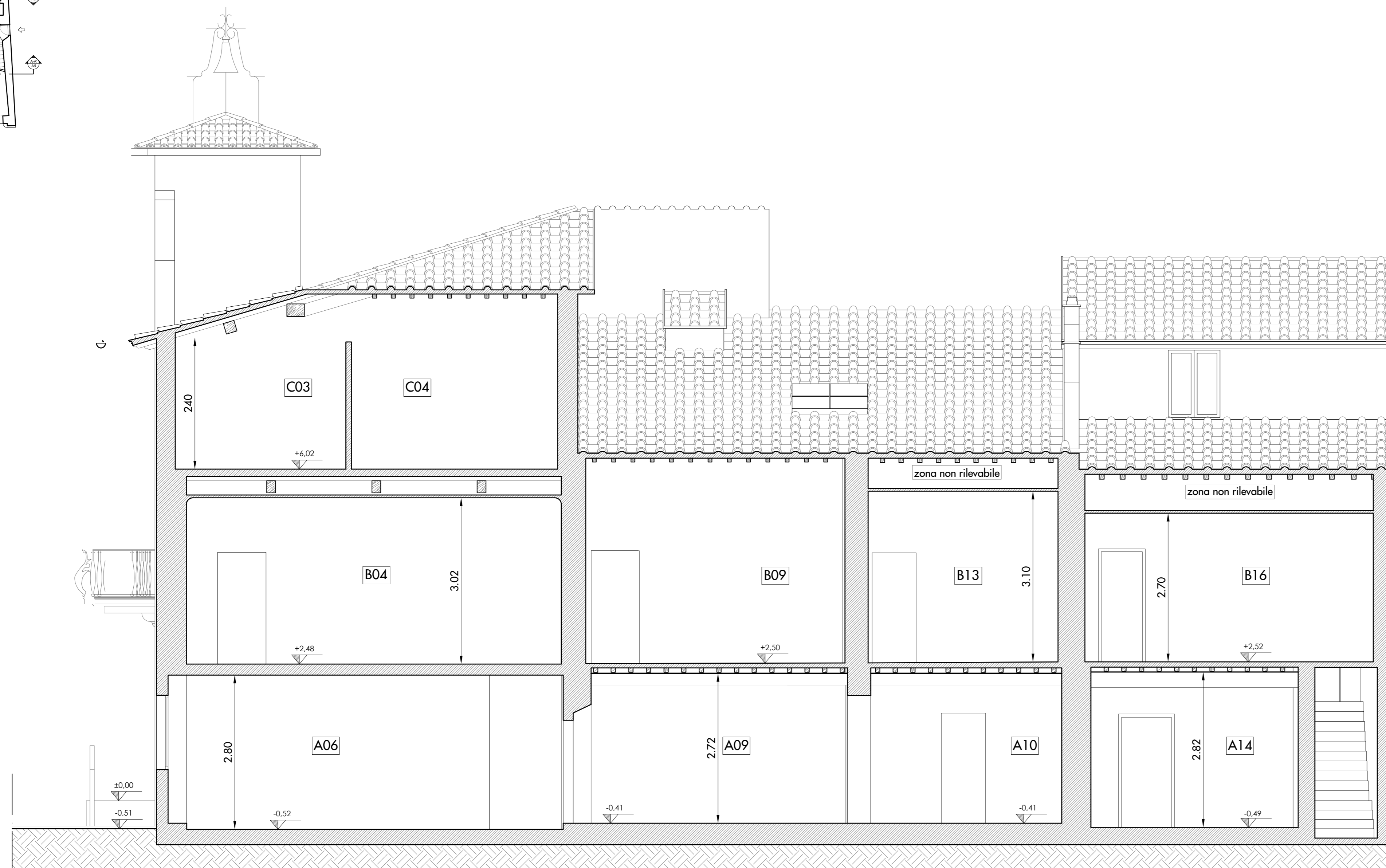
STATO ATTUALE - SEZIONE FF' SCALA 1:50
