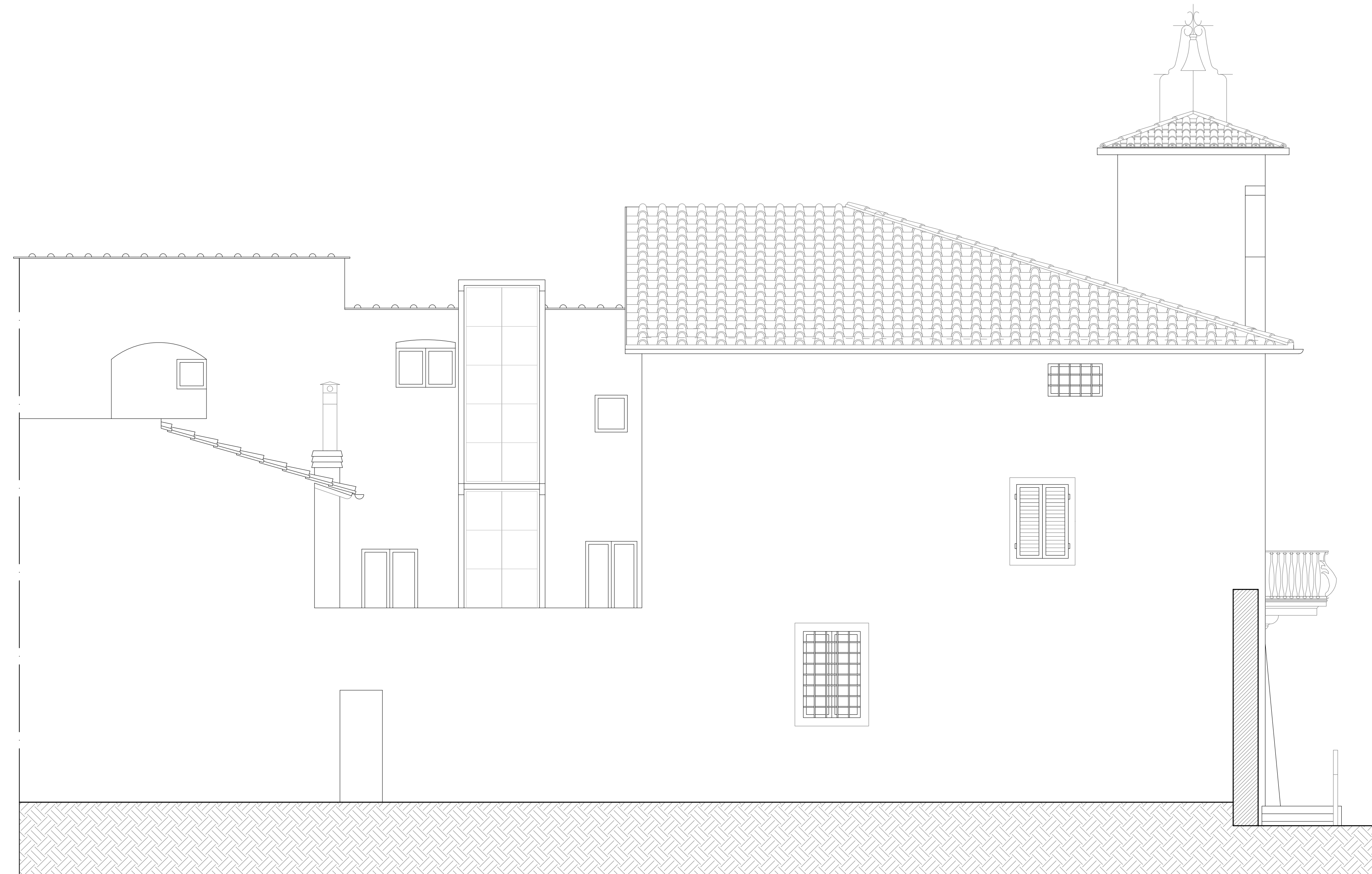
STATO DI PROGETTO - PROSPETTO NORD-EST SCALA 1:50
