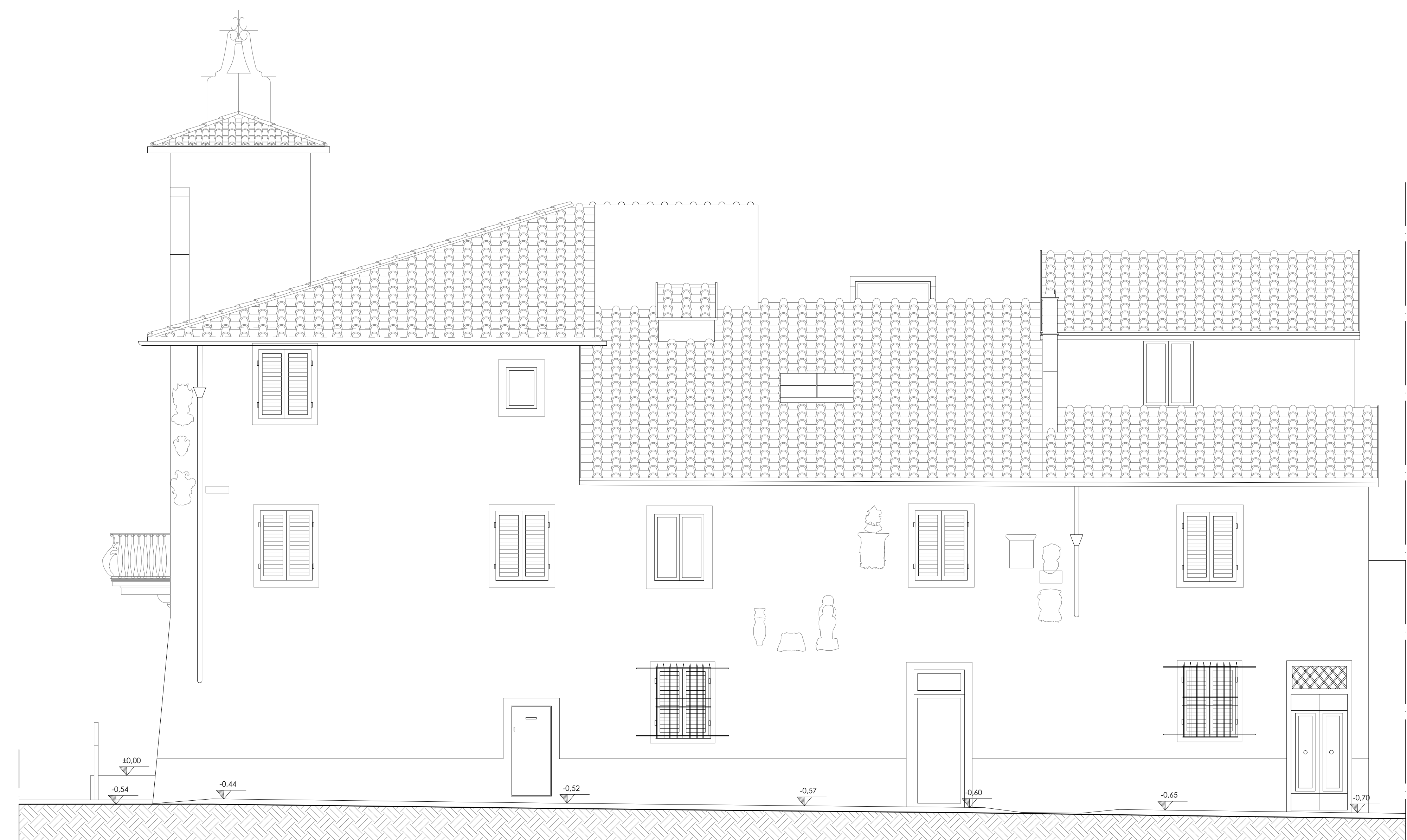
STATO DI PROGETTO - PROSPETTO SUD-OVEST SCALA 1:50
