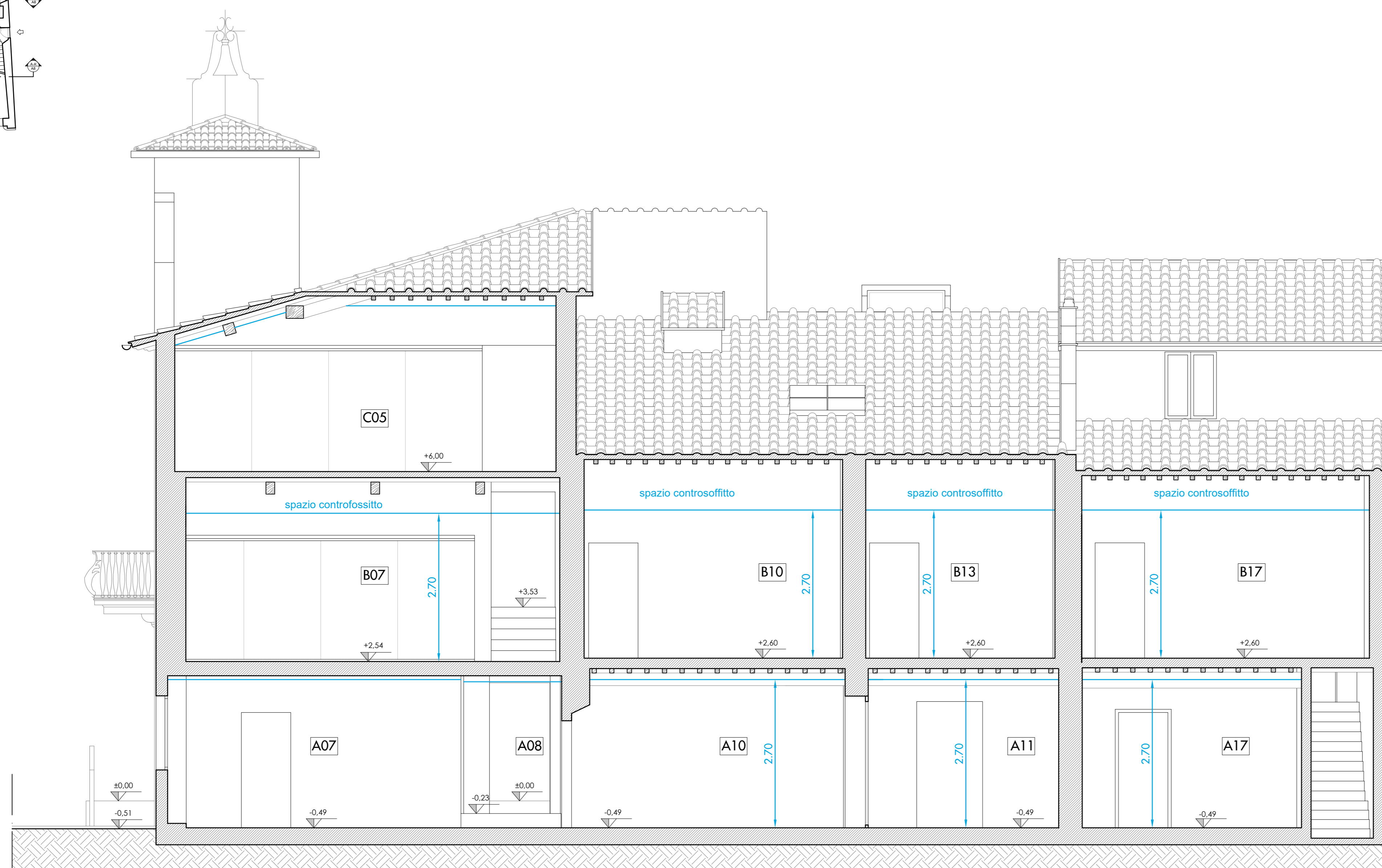
STATO DI PROGETTO - SEZIONE F-F' SCALA 1:50
