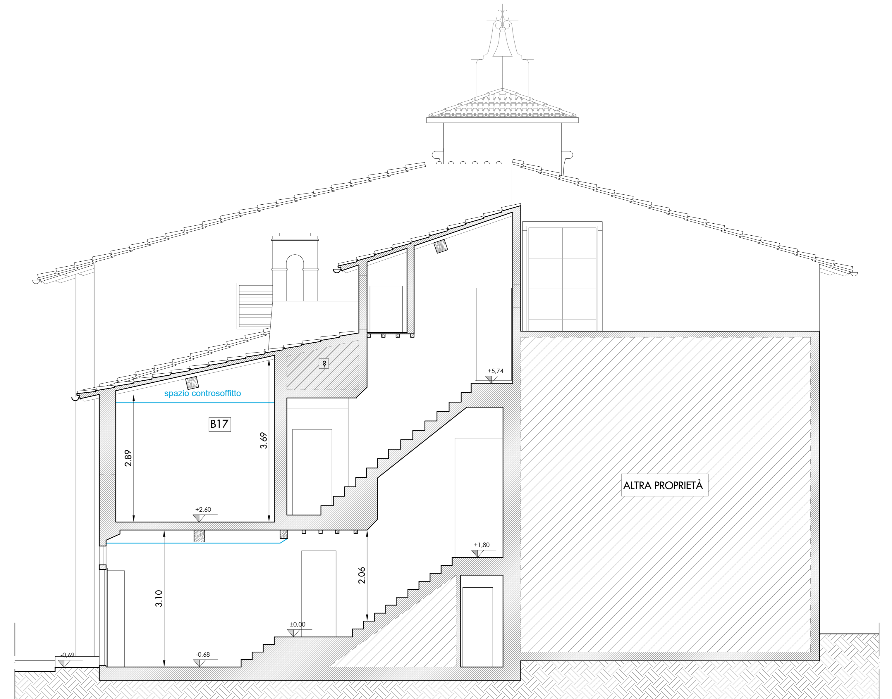
STATO ATTUALE - SEZIONE C-C' SCALA 1:50
