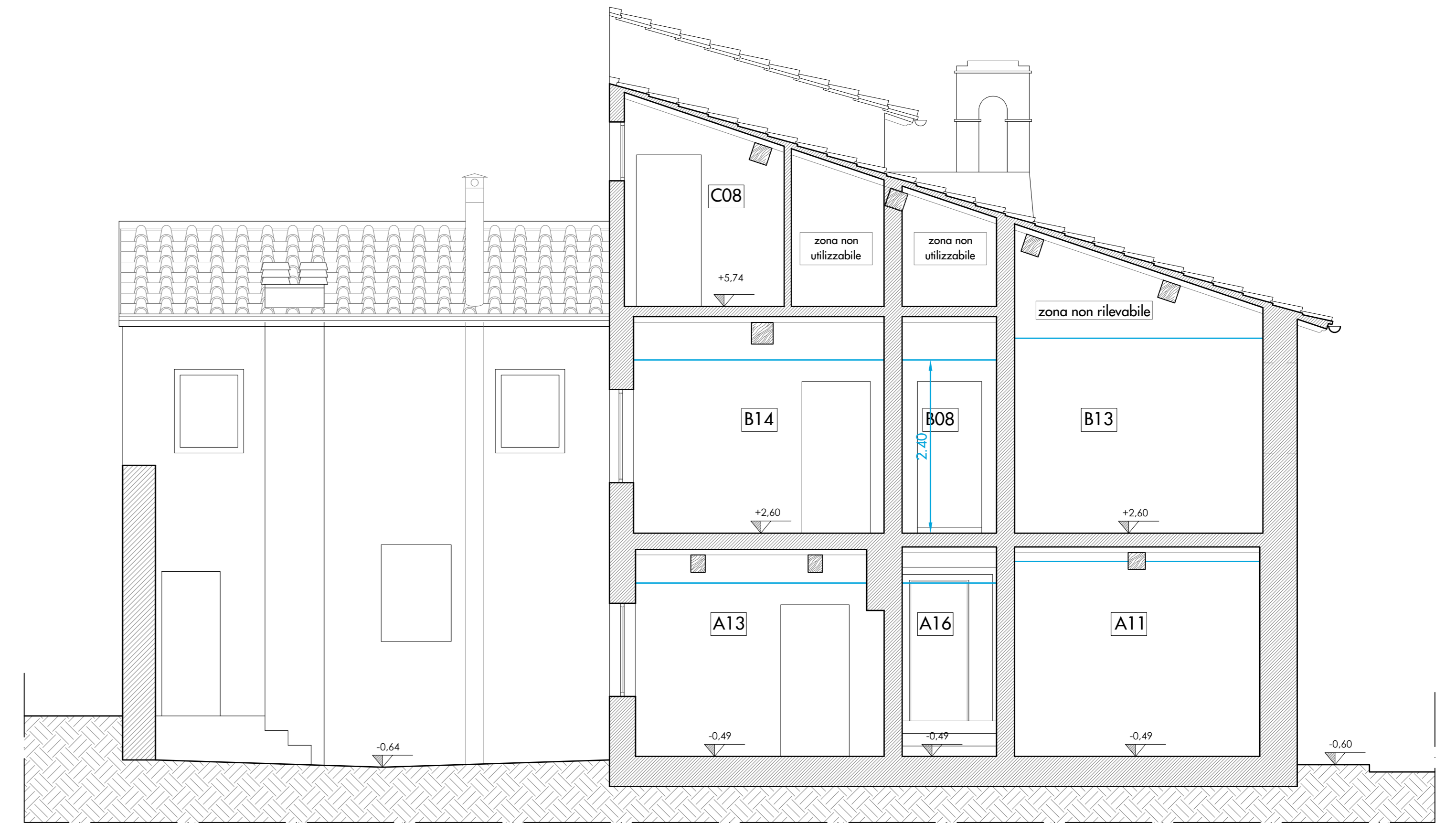
STATO DI PROGETTO - SEZIONE B-B' SCALA 1:50
