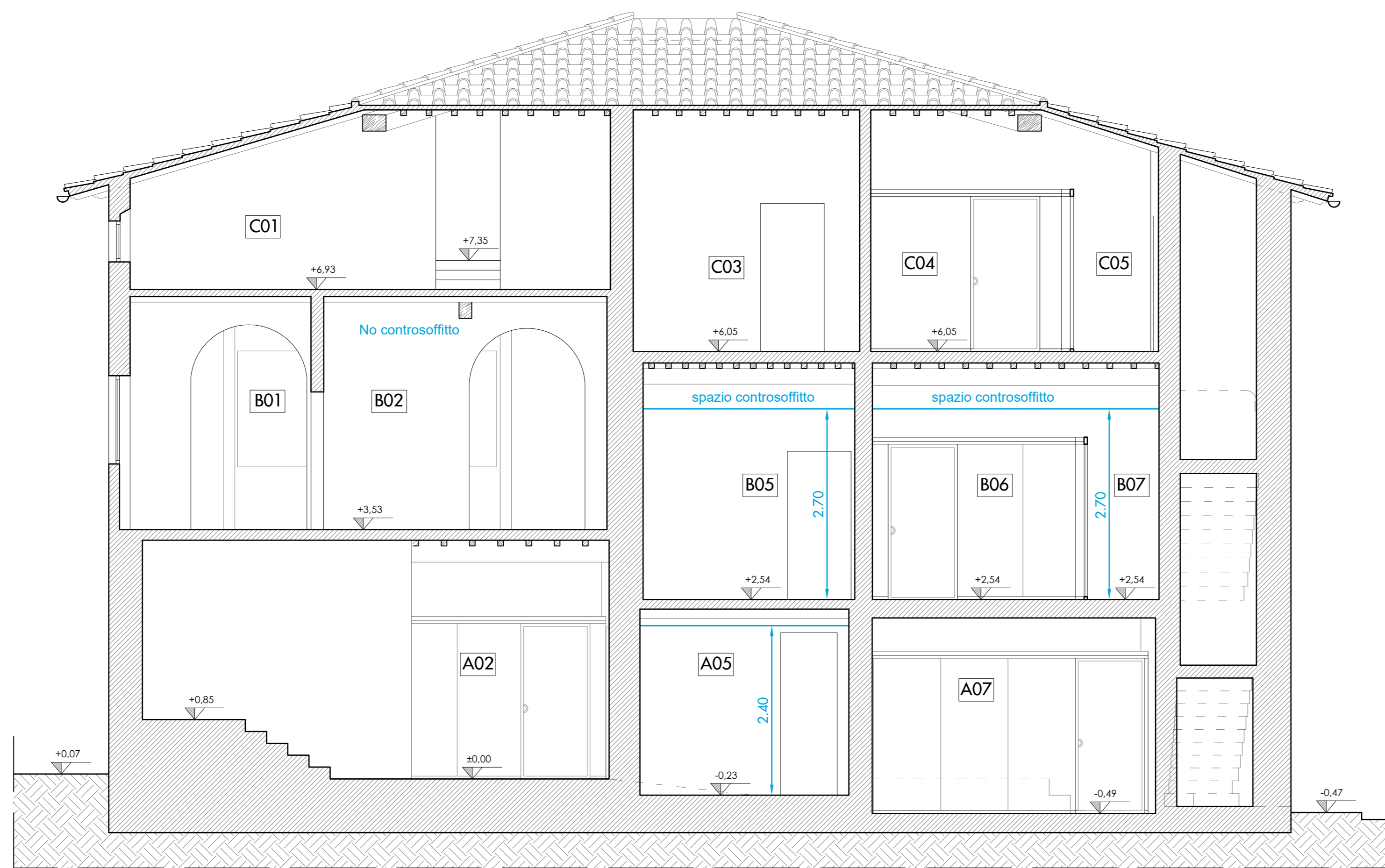
STATO DI PROGETTO - SEZIONE A-A' SCALA 1:50
