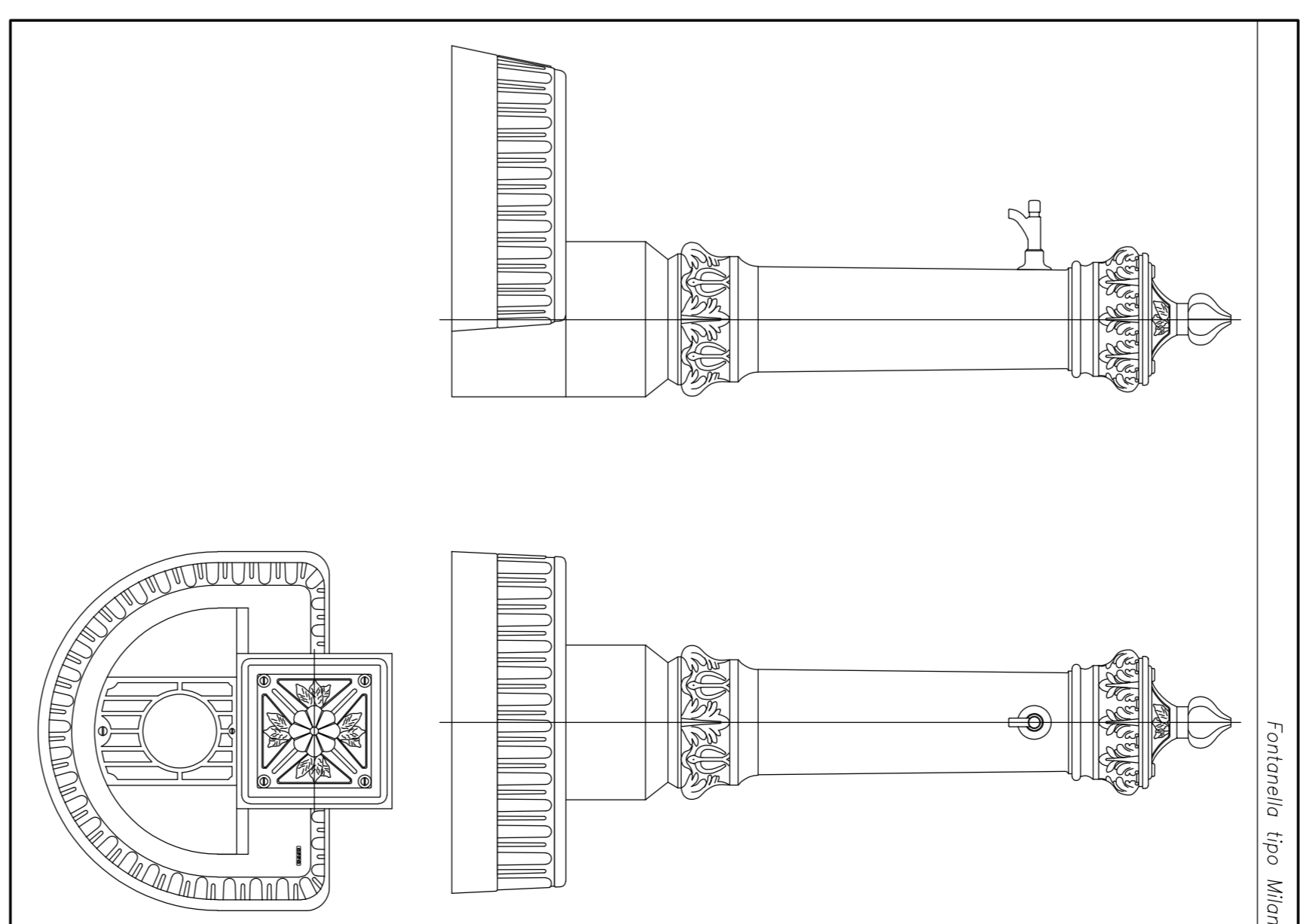
PARTICOLARI DELLA FONTANELLA
