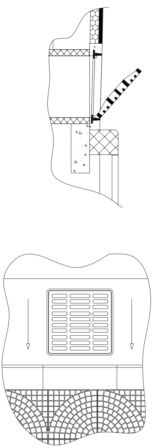
Cantierista stradale con griglia continua GS
