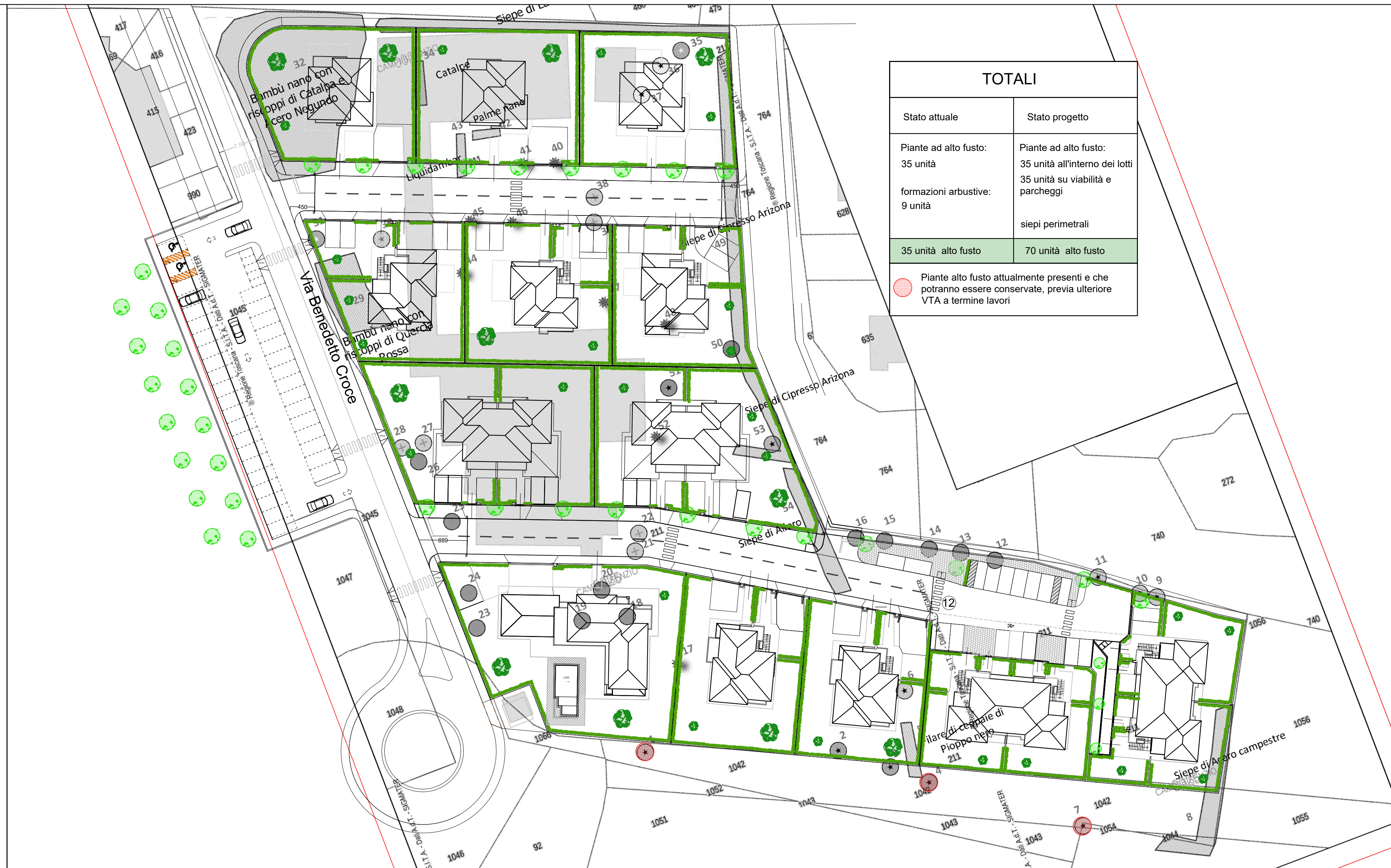
Planimetria sovrapposto Scala 1:500
