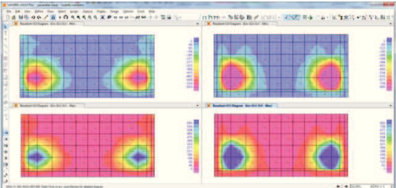
Sollecitazioni taglienti V13/V23 – ENV SLU-SLV (kN,m,C)
