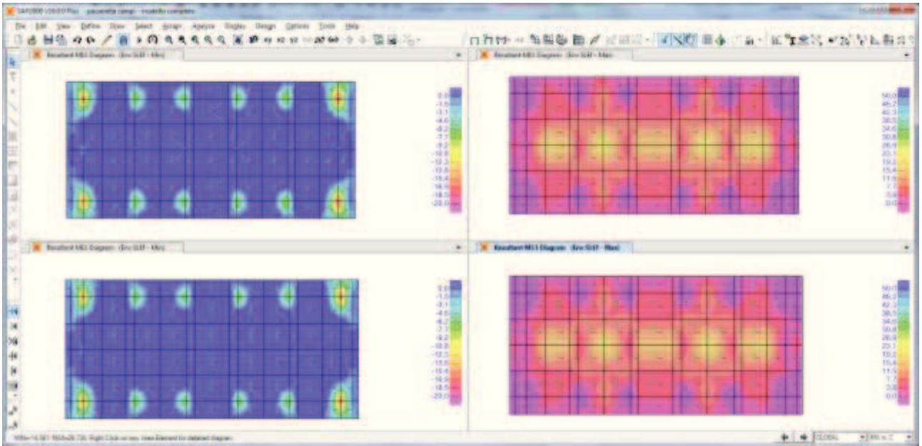
Sollecitazioni flettenti M11 – ENV_SLEf (kN,m,C)
