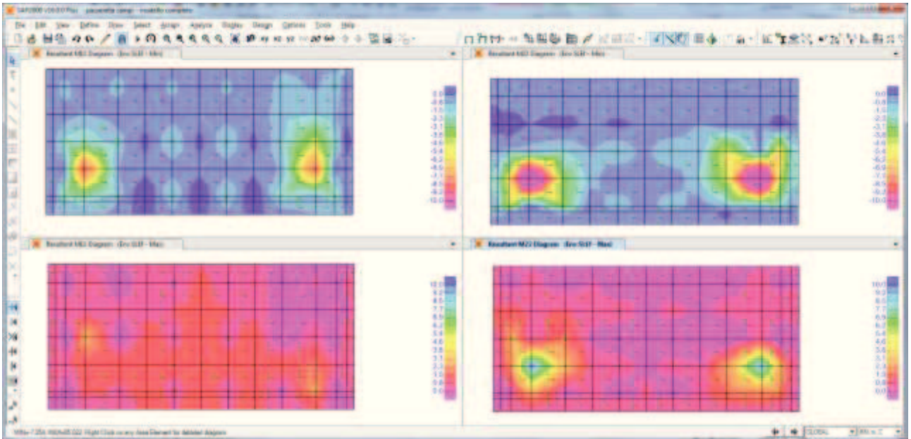
Sollecitazioni flettenti M11/M22 – ENV_SLEf (kN,m,C)
