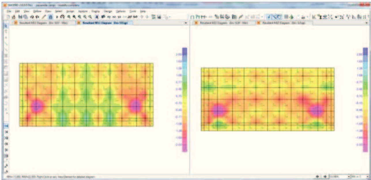
Sollecitazioni flettenti M11/M22 – SLE_qp (kN,m,C)
