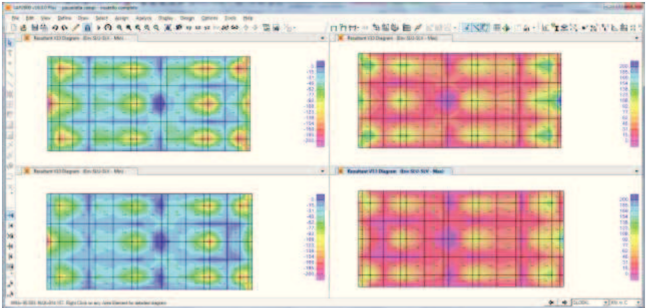
Sollecitazioni taglianti V13 – ENV SLU-SLV (kN,m,C)
