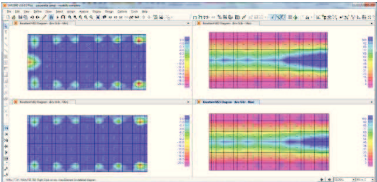
Sollecitazioni flettenti M22 – ENV_SLEr (kN,m,C)
