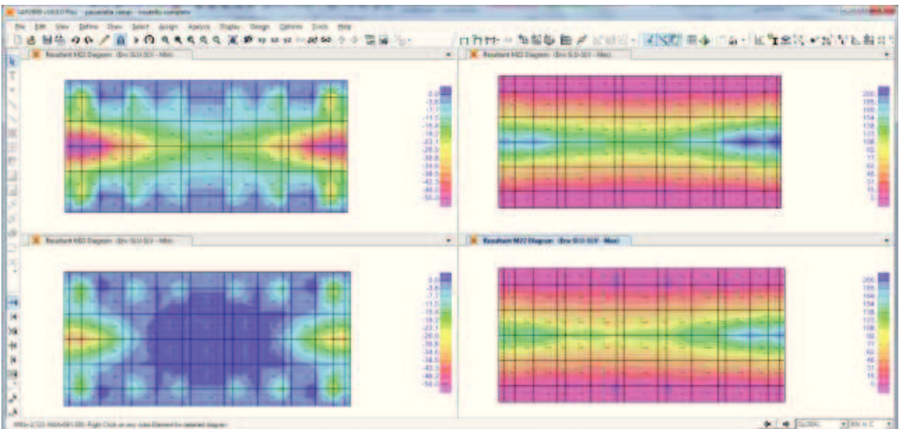
Sollecitazioni flettenti M22 – ENV SLU-SLV (kN,m,C)
