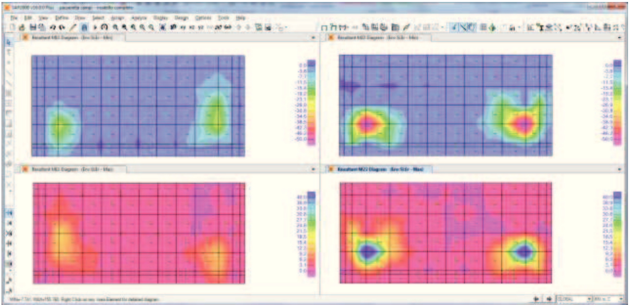
Sollecitazioni flettenti M11/M22 – ENV_SLEr (kN,m,C)
