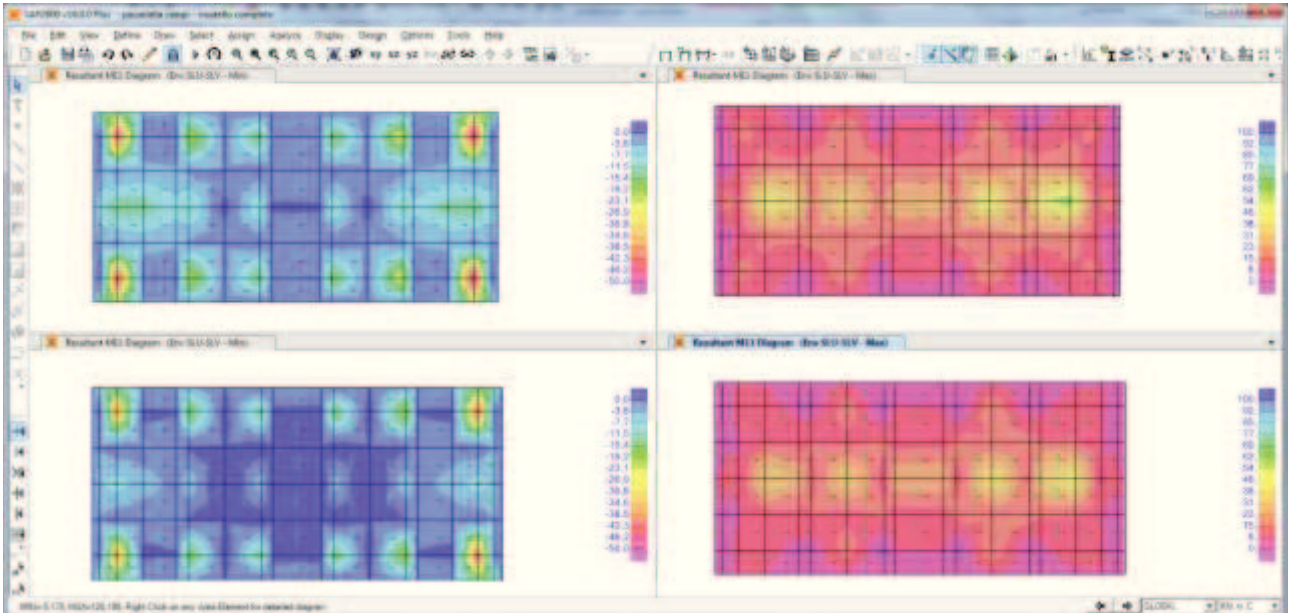
Sollecitazioni flettenti M11 – ENV SLU-SLV (kN,m,C)
