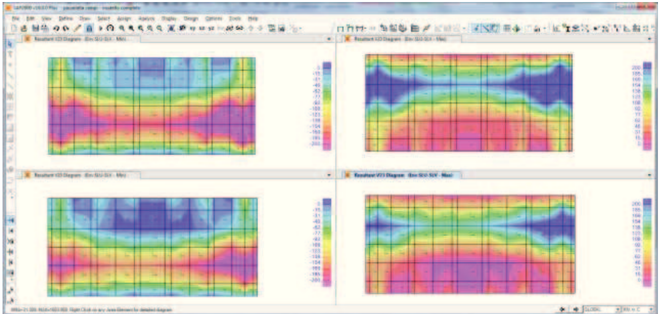
Sollecitazioni taglianti V23 – ENV SLU-SLV (kN,m,C)
