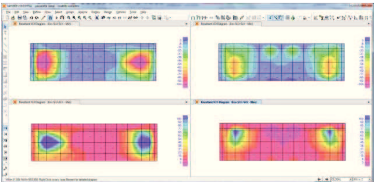
Sollecitazioni taglianti V13/V23 – ENV SLU-SLV (kN,m,C)
