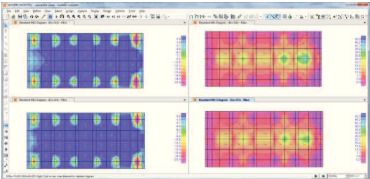
Sollecitazioni flettenti M11 – ENV_SLEr (kN,m,C)
