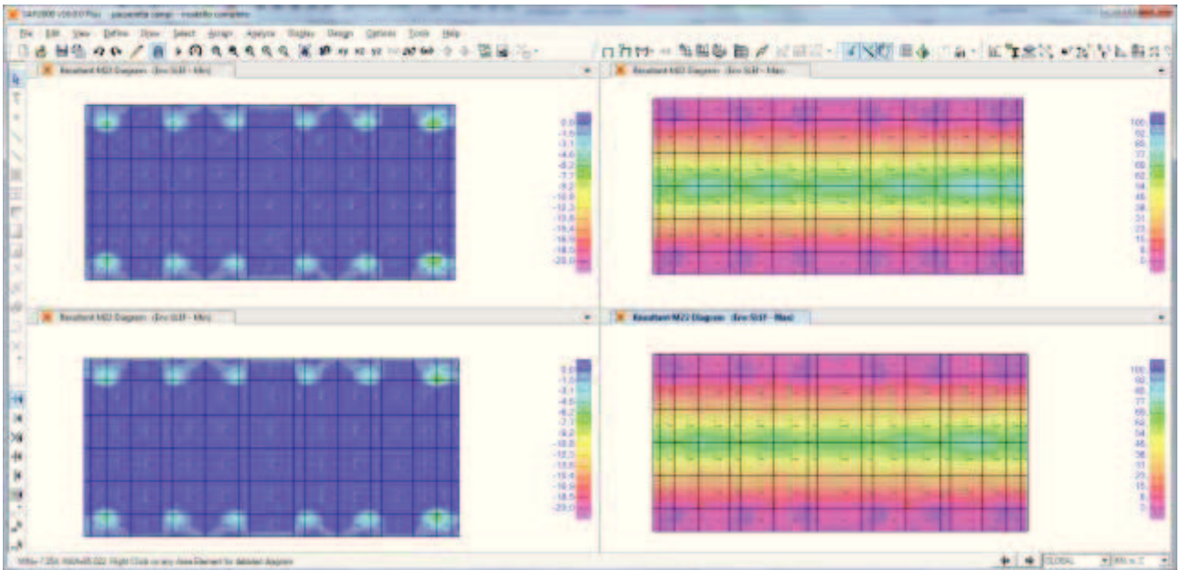
Sollecitazioni flettenti M22 – ENV_SLEf (kN,m,C)
