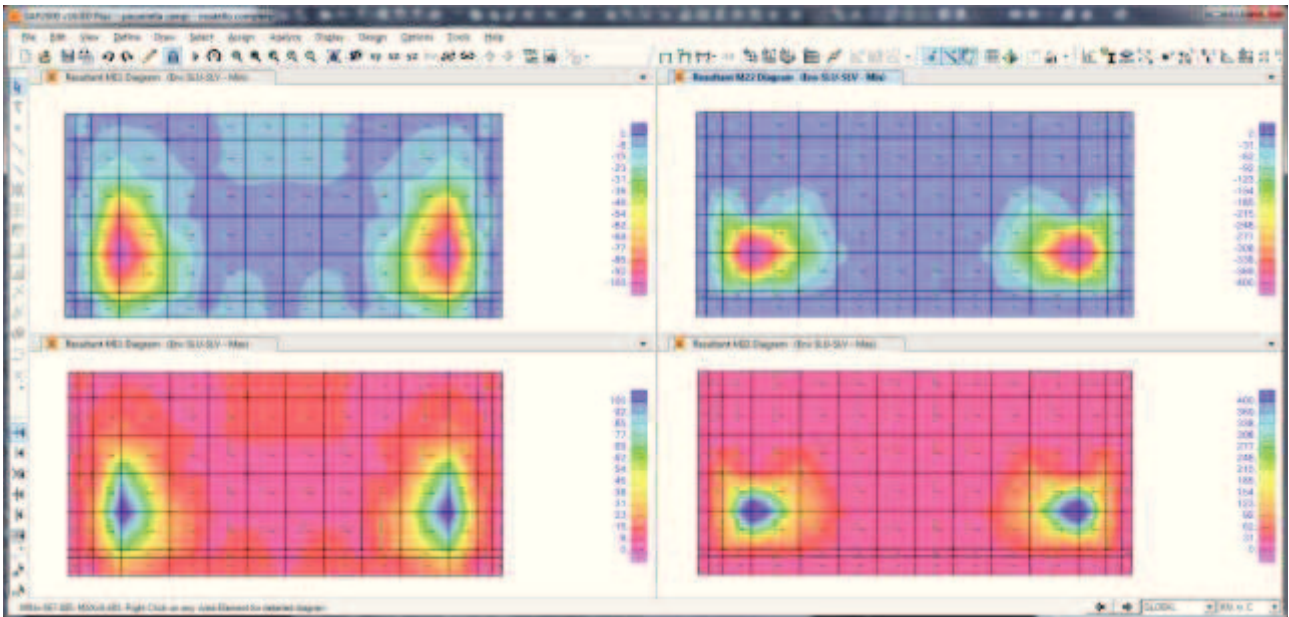
Sollecitazioni flettenti M11/M22 – ENV SLU-SLV (kN,m,C)
