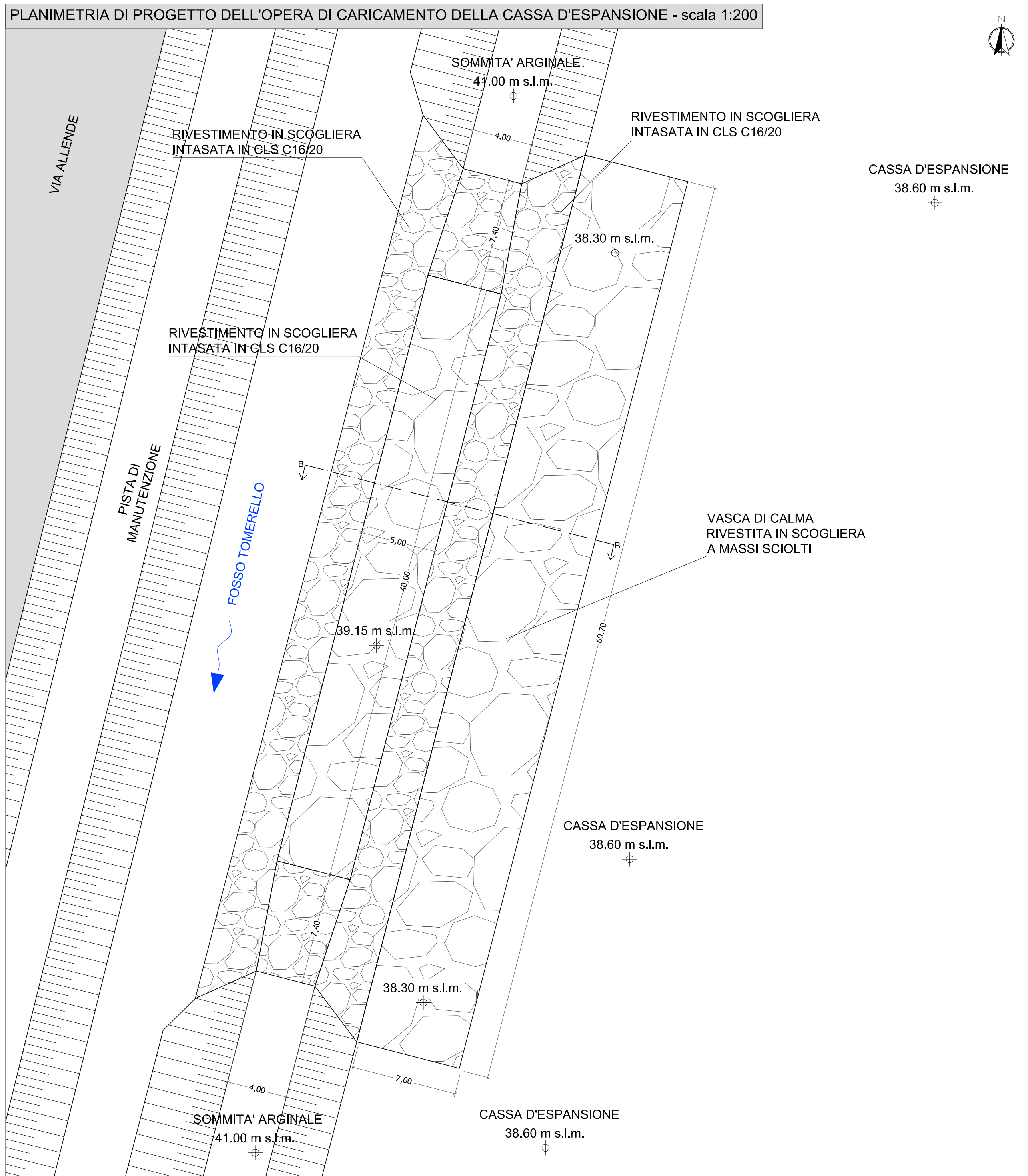
PLANIMETRIA DI PROGETTO DELL'OPERA DI CARICAMENTO DELLA CASSA D'ESPANSIONE - scala 1:200
