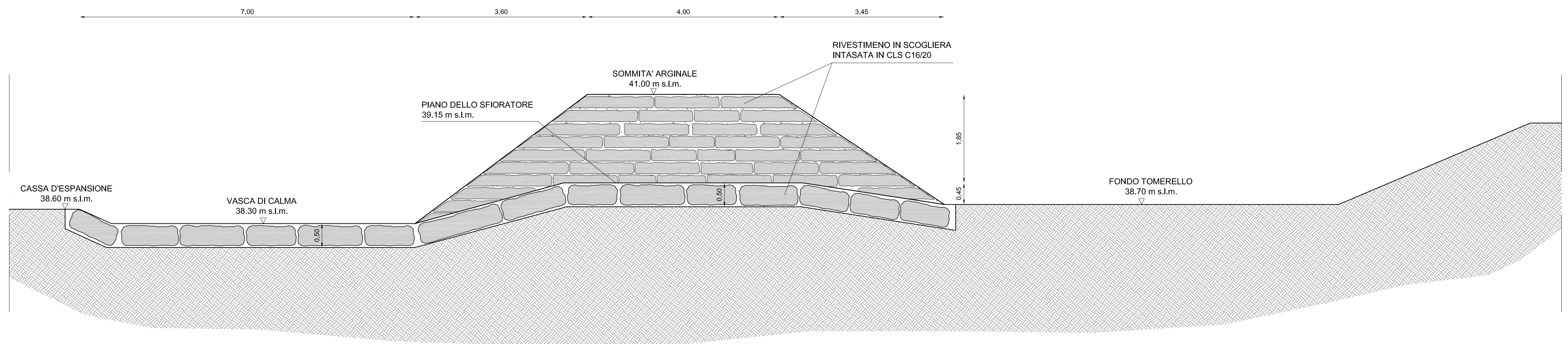
SEZIONE TIPO DEL RINGROSSO DELL'ARGINE SINISTRO DEL FOSSO TOMERELLO - scala 1:50
