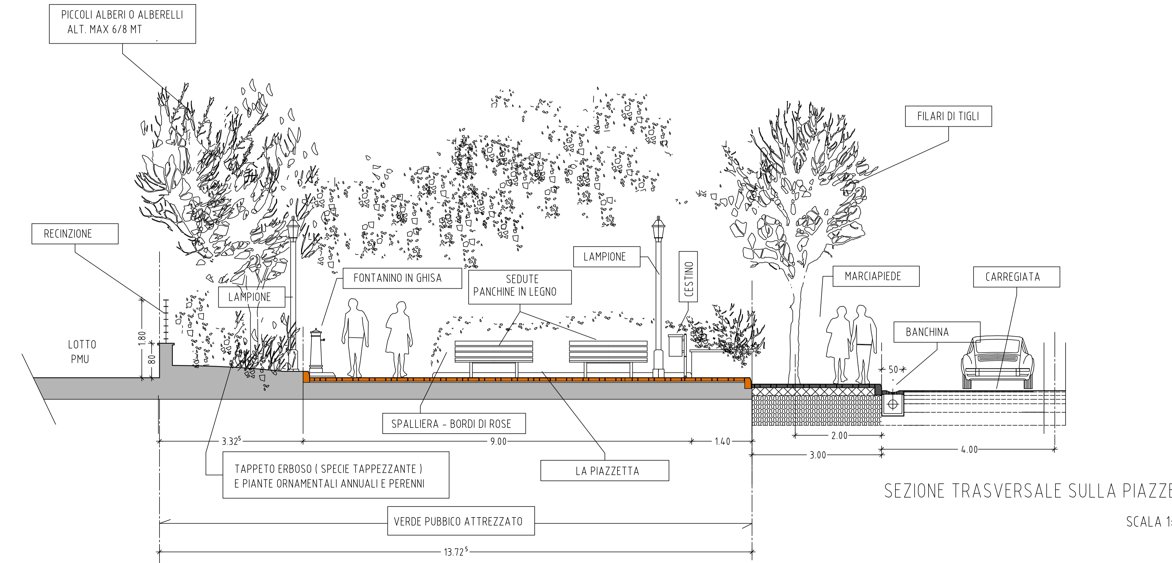
SEZIONE TRASVERSALE SUL PERCORSO INTERNO AL VERDE SCALA 1:50
